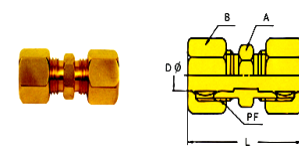
中間リングジョイント
