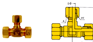
三方リングチーズ
