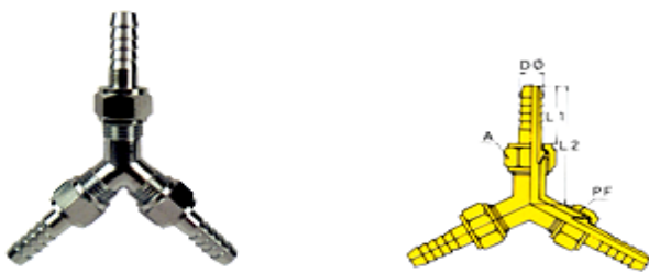
三方ホースジョイント
