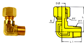
片口リングエルボ
